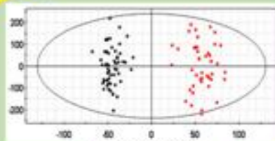
判別分析 (PLS)
